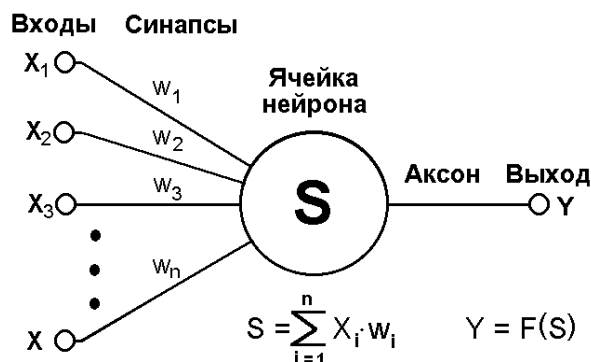
Рис. 1. Искусственный нейрон
